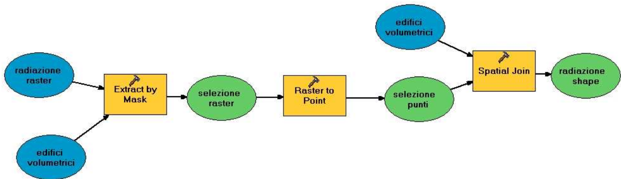
Figura 2 - Flusso delle operazioni attraverso il Model Builder
